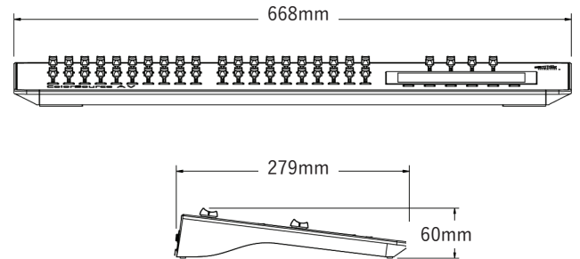
ColorSource 40 AV
